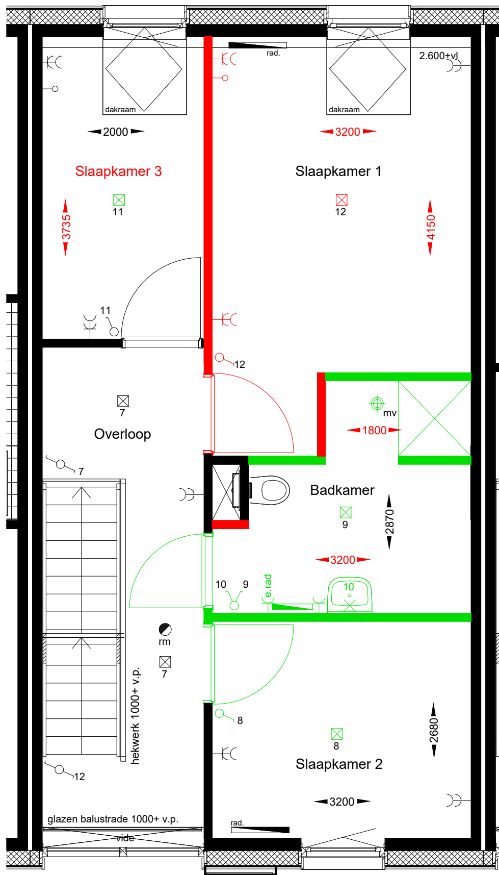
optie B38f: wijziging indeling 1e verdieping
